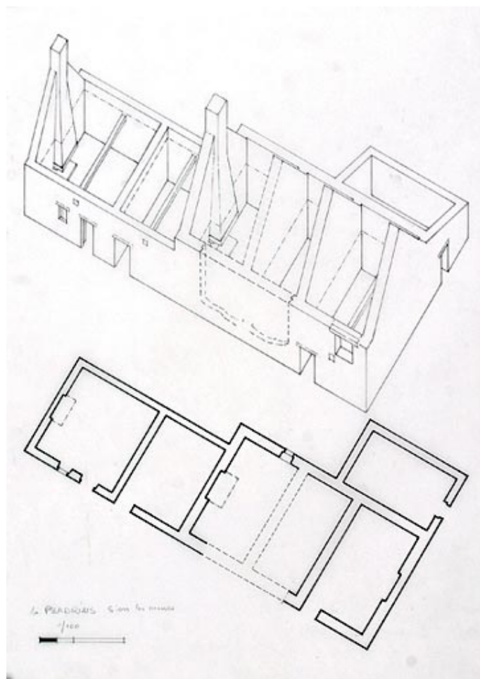
Fig. 10 - Sion-les-Mines, plan du petit alignement de la Perdriais qui comporte deux logis-étable du XIXe siècle et un ancien logis du XVIIIe siècle transformé en étable. Photo Bernard Renoux, droits réservés.
