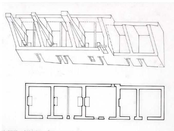
Fig. 8 - Sion-les-Mines, plan de l'alignement composé de cinq logis, XVIIIe et XIXe siècle. Photo Bernard Renoux, droits réservés.
